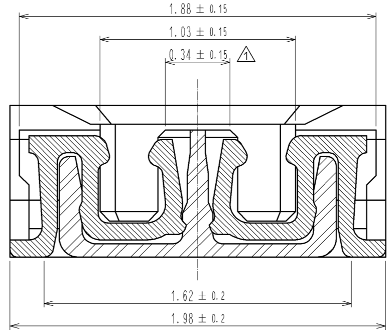
A-A (50:1)
