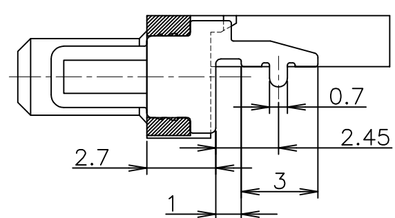
A-A SCALE 5:1
