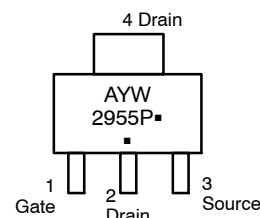
SOT-223 CASE 318E STYLE 3
