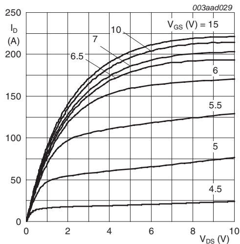
T_j = 25\text{ °C} ; t_p = 300\mu\text{s}
