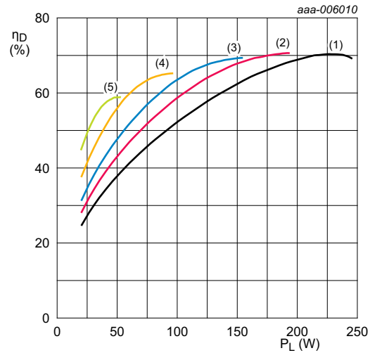
I_{Dq} = 100 \text{ mA}; f = 1300 \text{ MHz}. (1) V_{DS} = 32 \text{ V} (2) V_{DS} = 28 \text{ V} (3) V_{DS} = 25 \text{ V} (4) V_{DS} = 20 \text{ V} (5) V_{DS} = 15 \text{ V}
